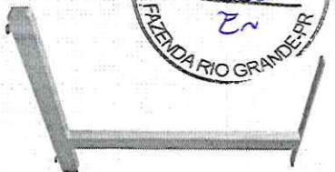
Standard EST-C1 | 590 X 710 Base 30x50 Coluna 30x30 Superior barra chata
